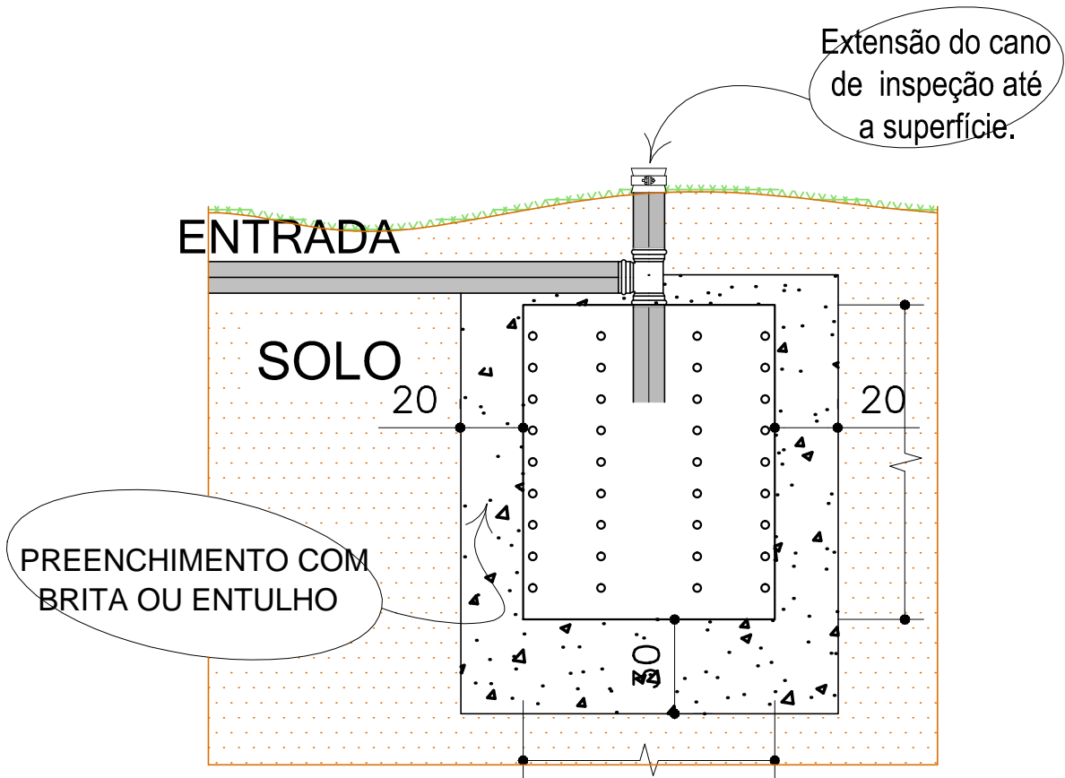
VISTA LATERAL
