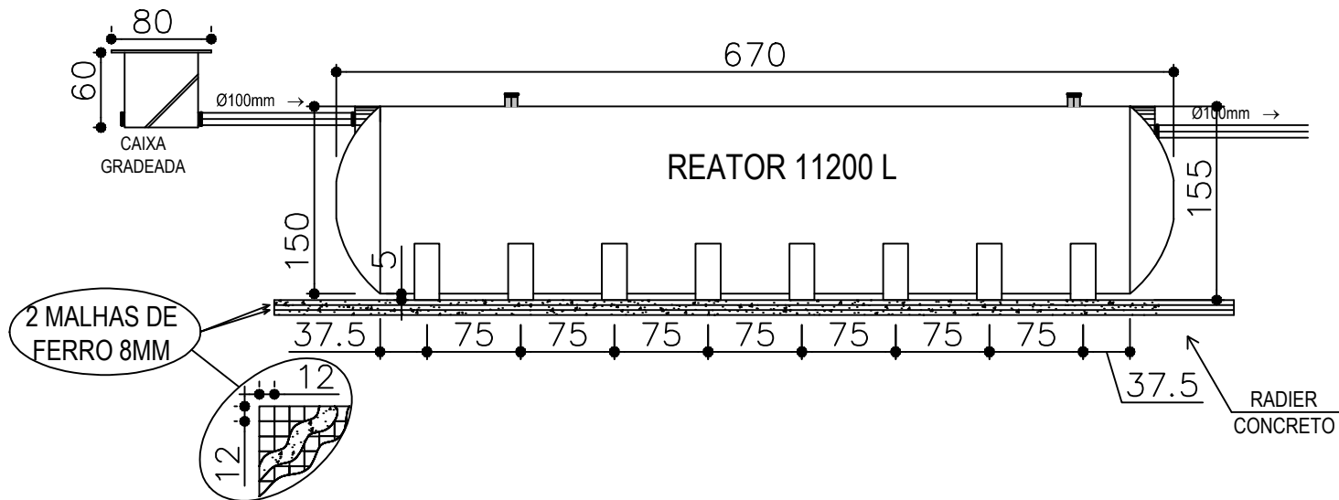
VISTA LATERAL
