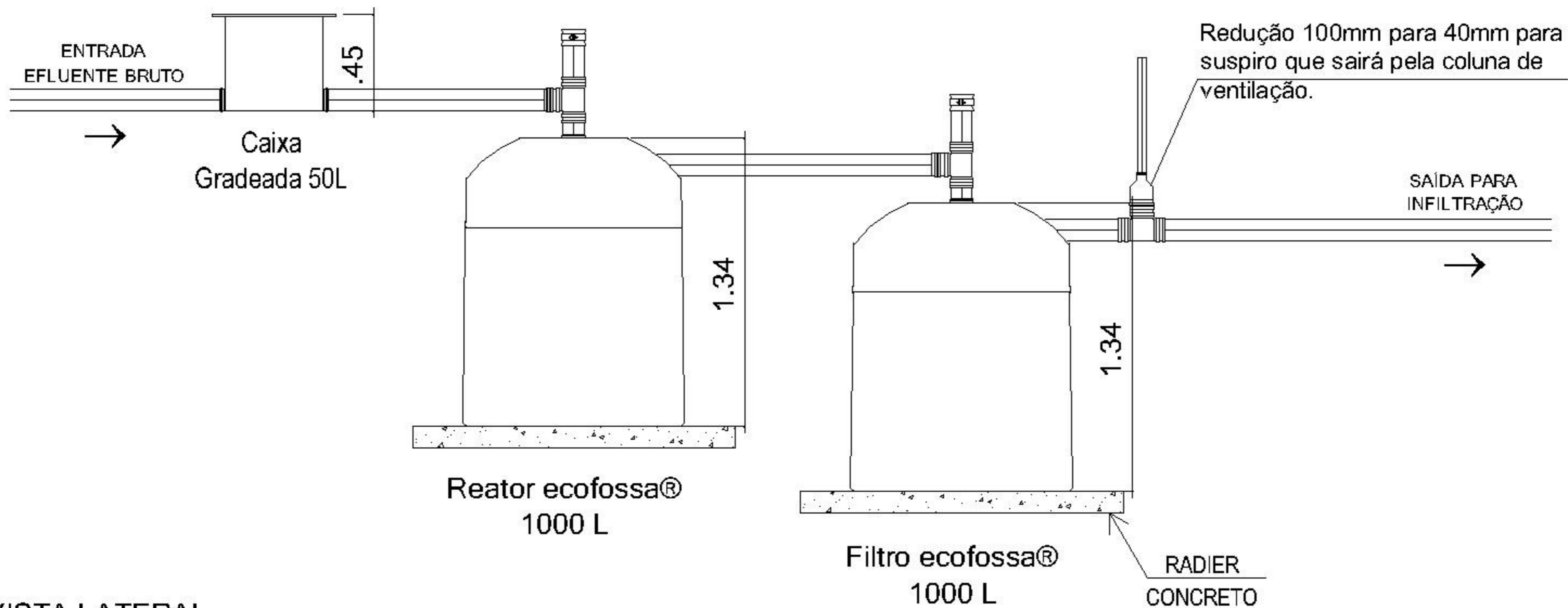
VISTA LATERAL
