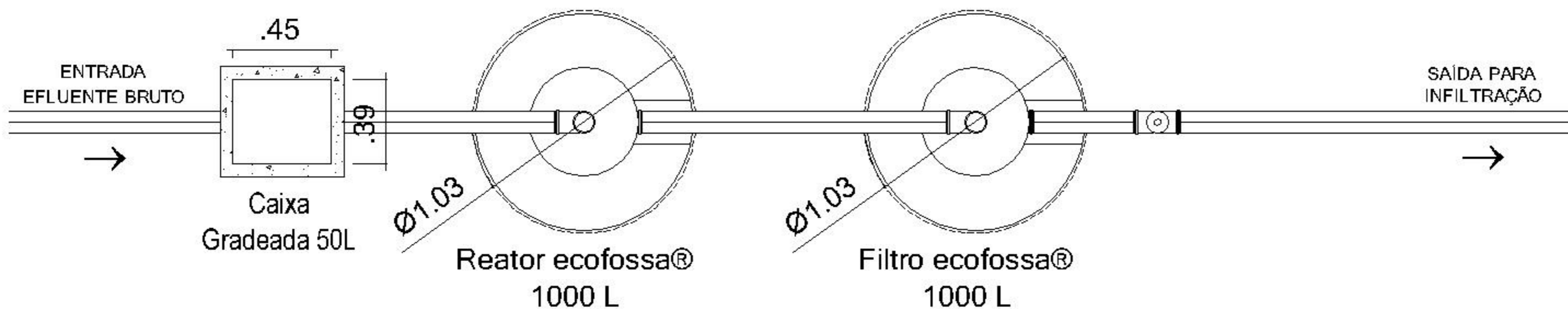
VISTA SUPERIOR
