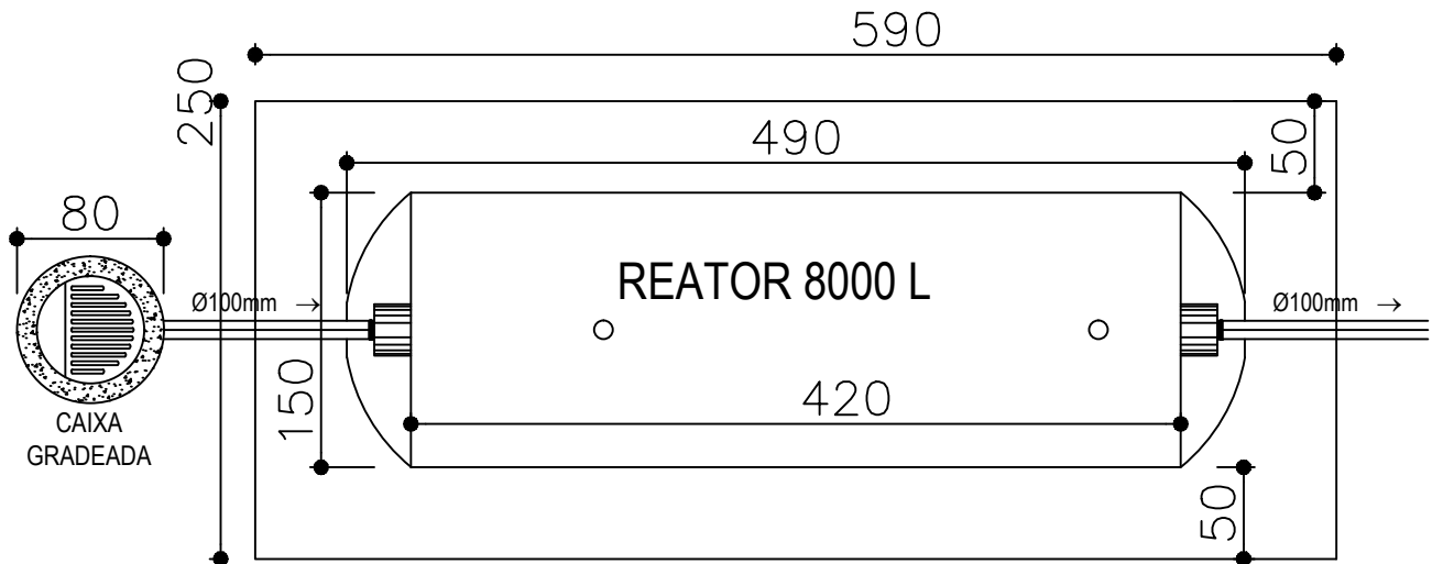
VISTA SUPERIOR
