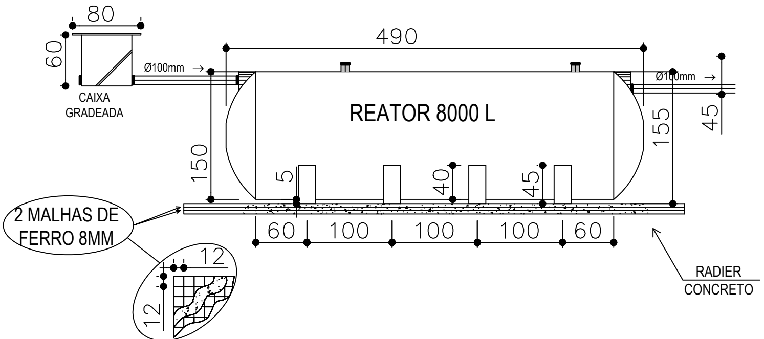
VISTA LATERAL
